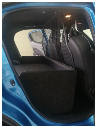
Kit VU avec grille arrêt de charge
